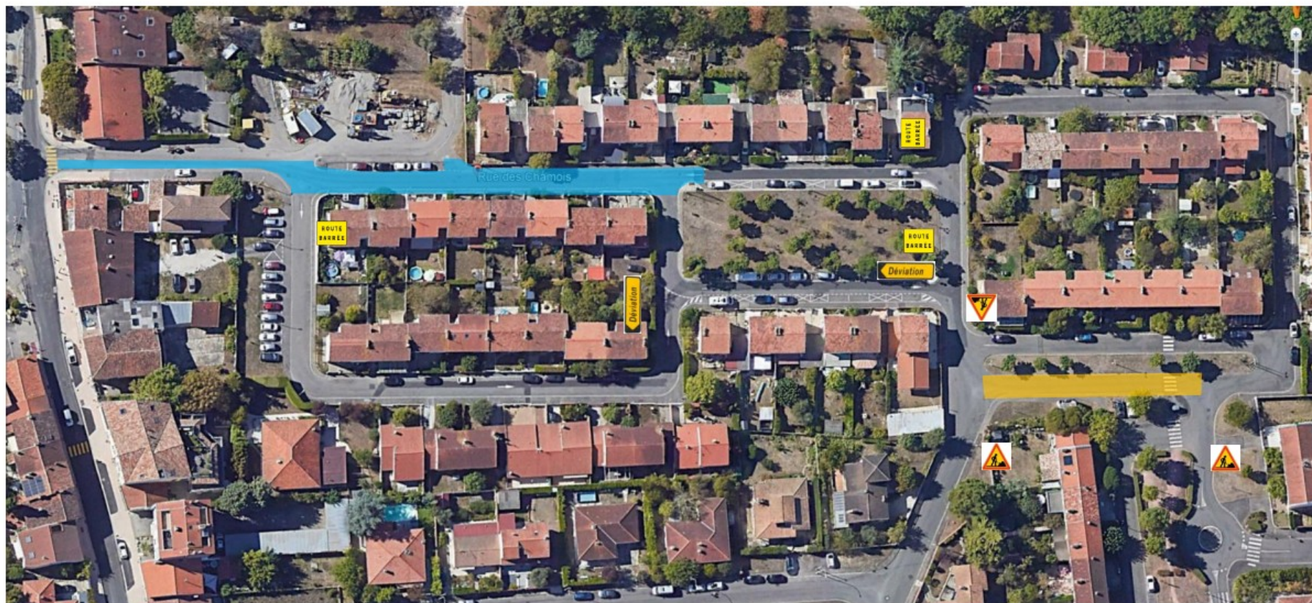
S04 (A) – Reprise Collecteur EU Chevreuils (DN250) + Voirie Chamois
